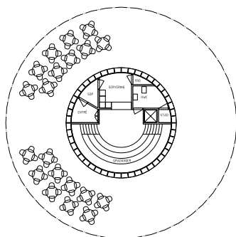
Bottenvåning med entré, servering och funktionsutrymmen.
