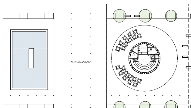
Bottenplan med Kungsgatan och "Likkistan", entré och uteservering mot väster.
